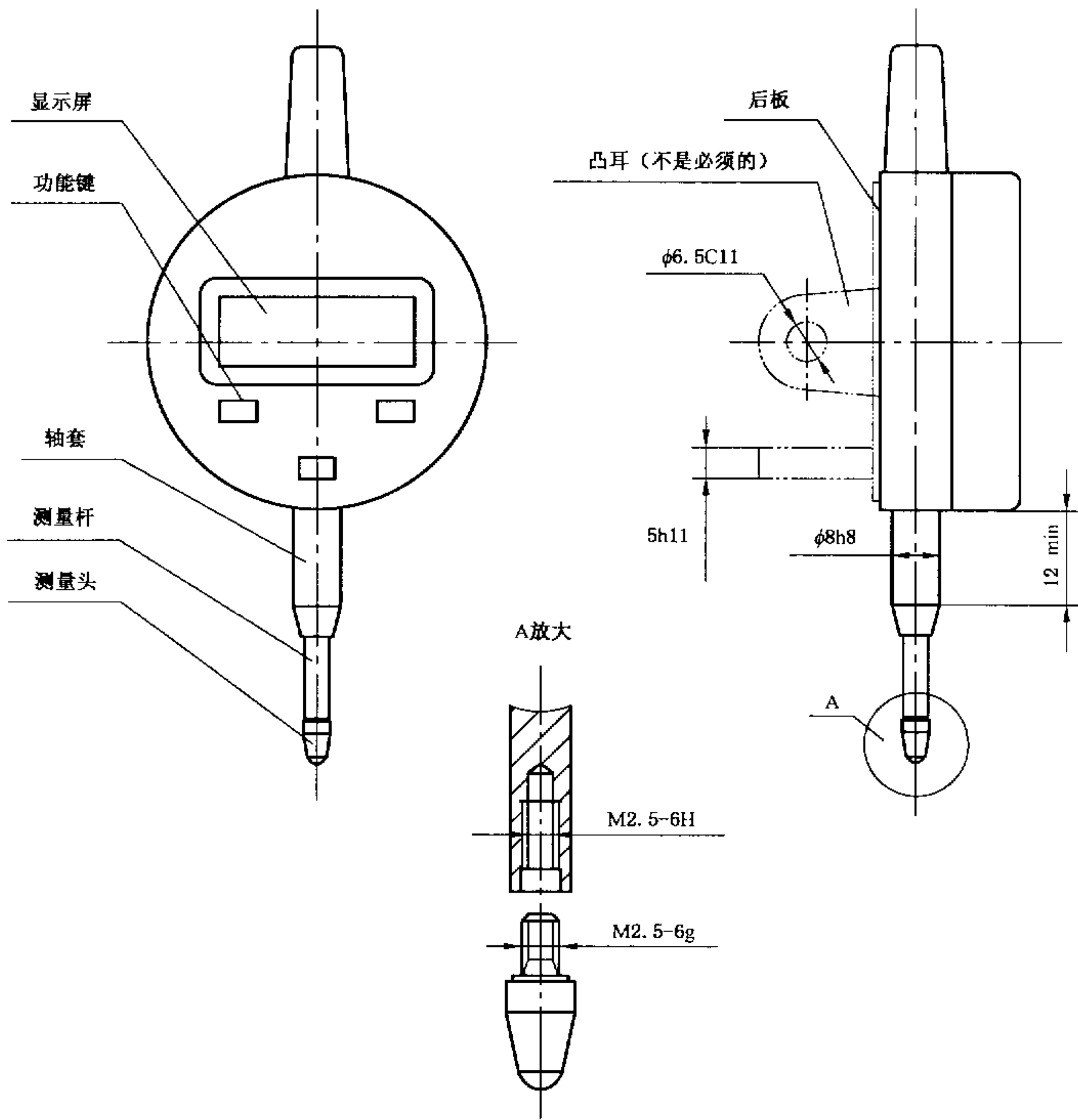
图 1 电子数显指示表的型式示意图
